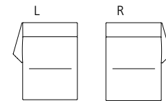
630-15 ARA B 145 T 175 H 78 SH 43 ST 137
