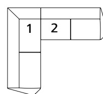
630-Version F B 288 T 266 H 78 SH 43
