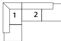
630-Version B B 280 T 200 H 78 SH 43
