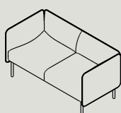
AL2 W 1460 D 730 H 700 S 440
