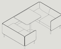
ALBT4-2335-ARM W 2335 D 1460 H 700 S 440
