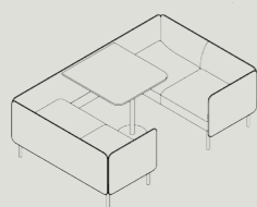
ALBT4-2185-ARM W 2185 D 1460 H 700 S 440
