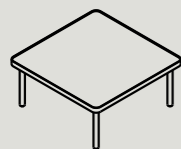
AT-310-A W 675 D 675 H 310 W 26.6" D 26.6" H 12.2"
