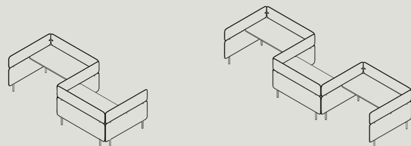
AWM-SPL2-A-XXXX 1330 - W 2855 / D 1460 / H 1025 1520 - W 3235 / D 1460 / H 1025 1710 - W 3615 / D 1460 / H 1025
