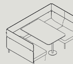
AMBT4-2335-NA W 2335 D 1410 H 1025 S 440
