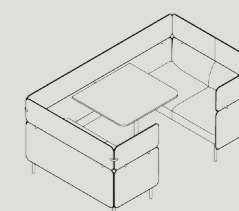
AMBT4-2335-ARM W 2335 D 1460 H 1025 S 440
