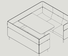
AMBT6-2335-ARM W 2335 D 2140 H 1025 S 440
