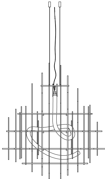
LATO | SIDE
