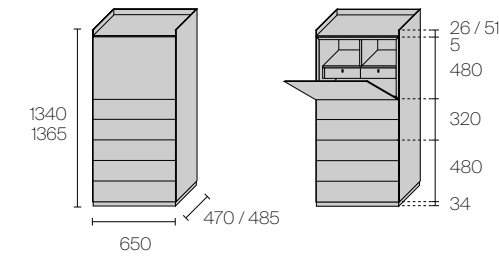
Self bold
